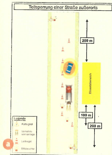
Teilsperre (Absicherung) einer Landstraße
