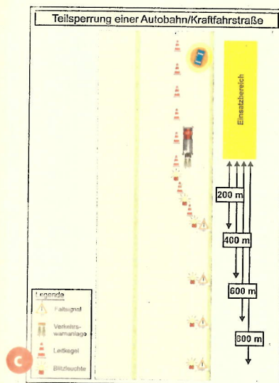
Teilsperre (Absicherung) einer Autobahn
