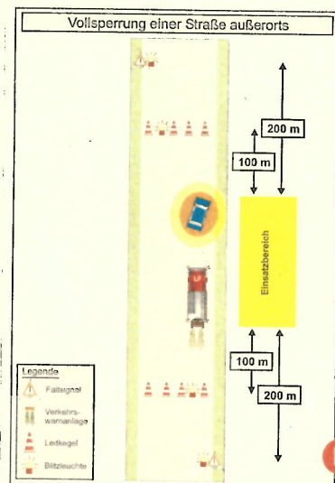
Vollsperrung einer Landstraße
