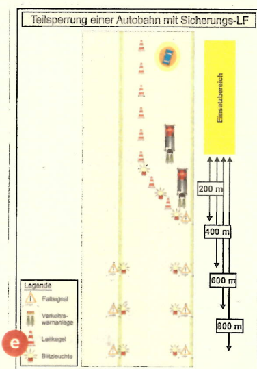
Teilsperre Autobahn mit Sicherungs-LF
