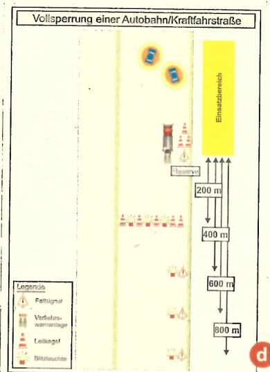
Vollsperrung einer dreispurigen Autobahn
